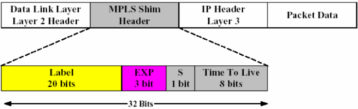
Fig. 1. MPLS shim header
